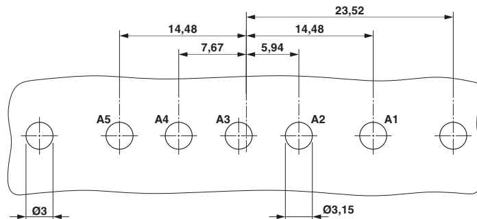
Otworowanie/geometria płytek lutowniczych
