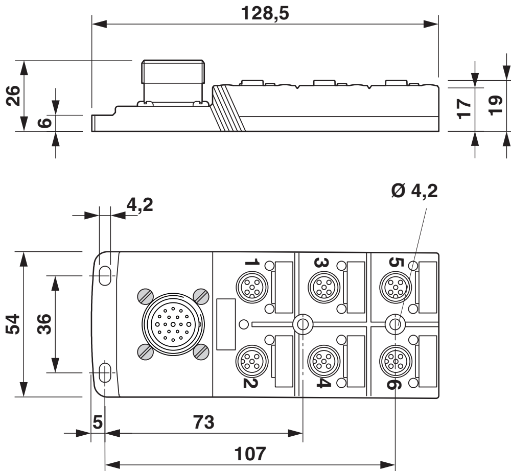
Rysunek wymiarowy
