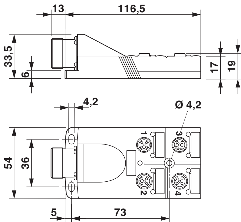
Rysunek wymiarowy
