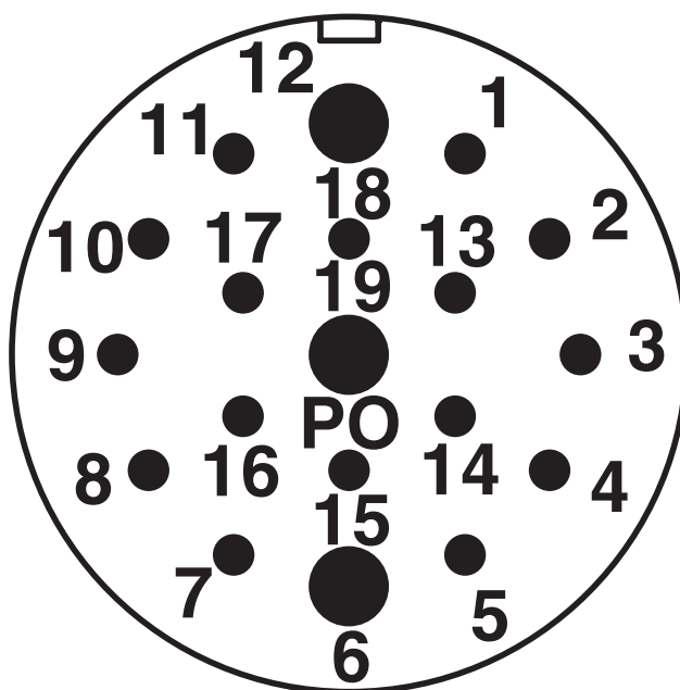
Rysunek schematyczny
