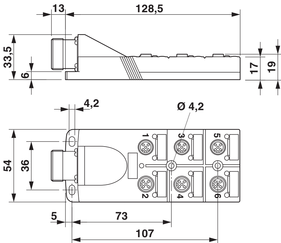
Rysunek wymiarowy
