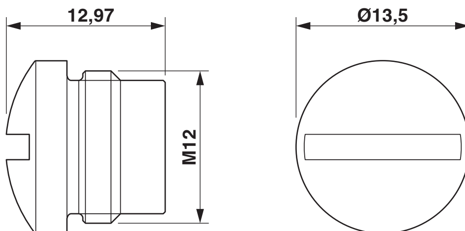
Rysunek wymiarowy
