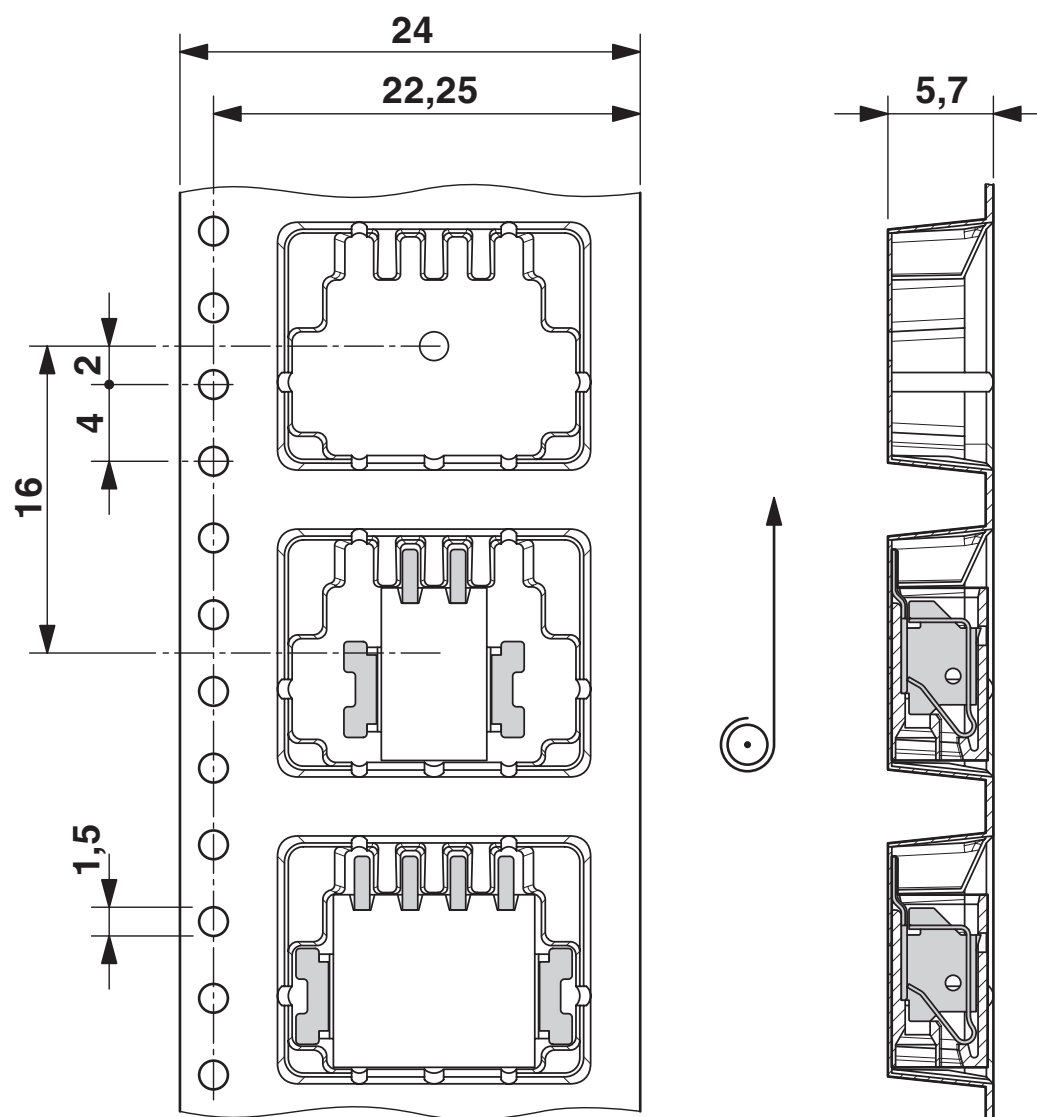
Rysunek wymiarowy
