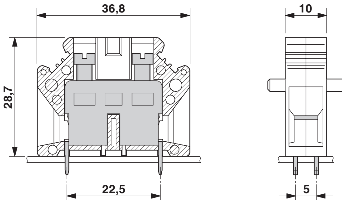
Rysunek wymiarowy
