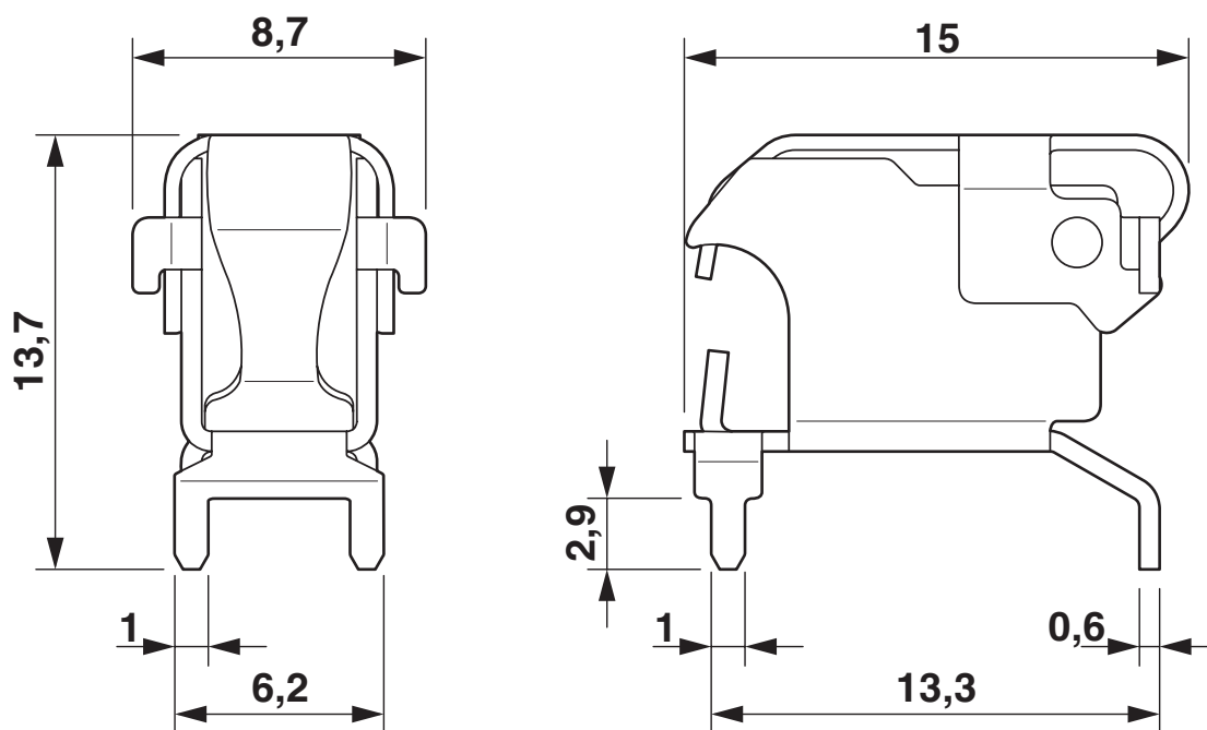
Rysunek wymiarowy
