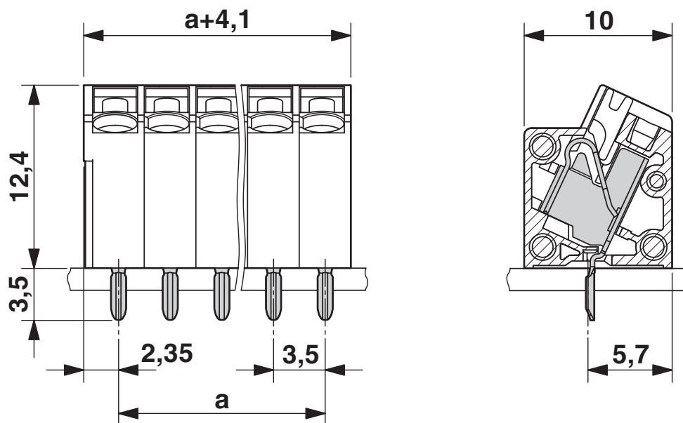
Rysunek wymiarowy
