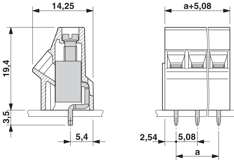
Rysunek wymiarowy
