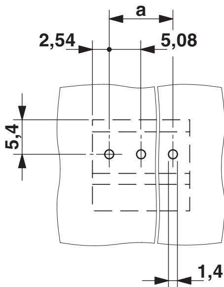
Otworowanie/geometria płytek lutowniczych
