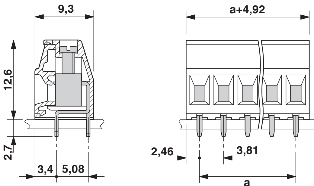
Rysunek wymiarowy
