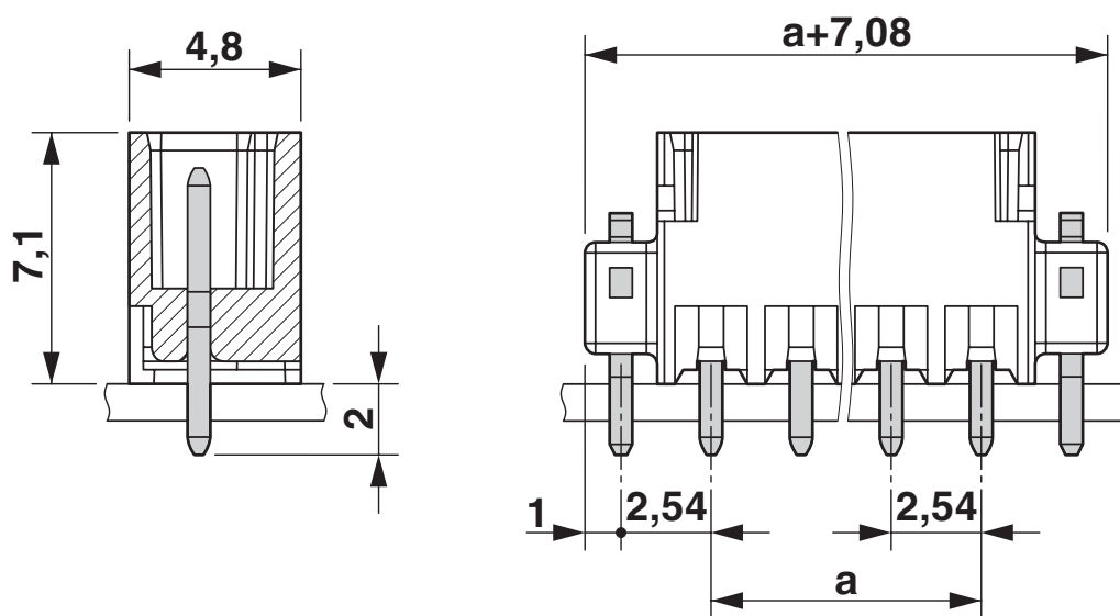
Rysunek wymiarowy
