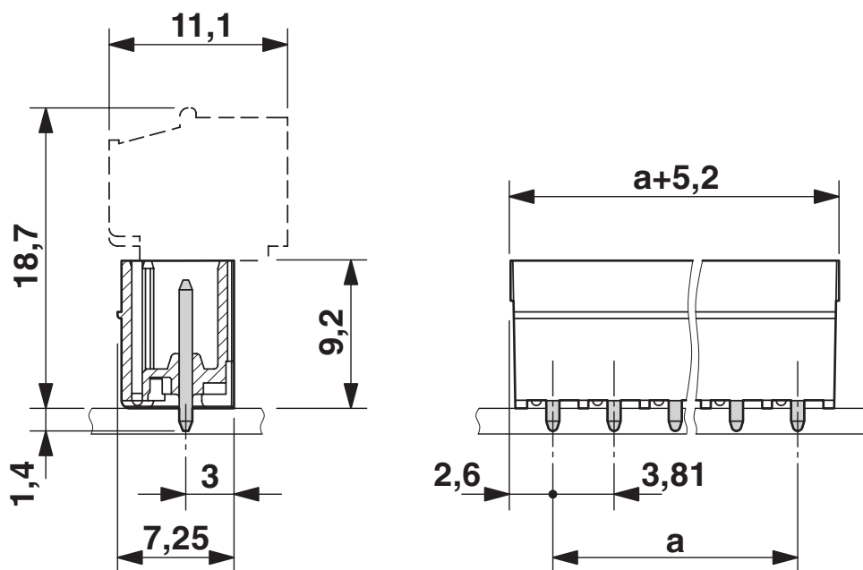
Rysunek wymiarowy
