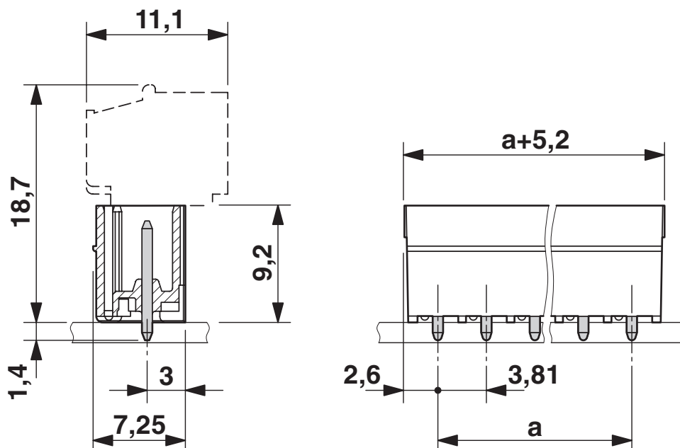
Rysunek wymiarowy
