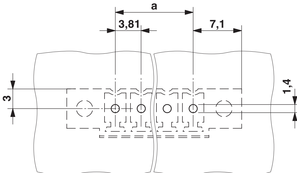
Otworowanie/geometria płytek lutowicznych
