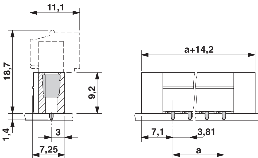
Rysunek wymiarowy
