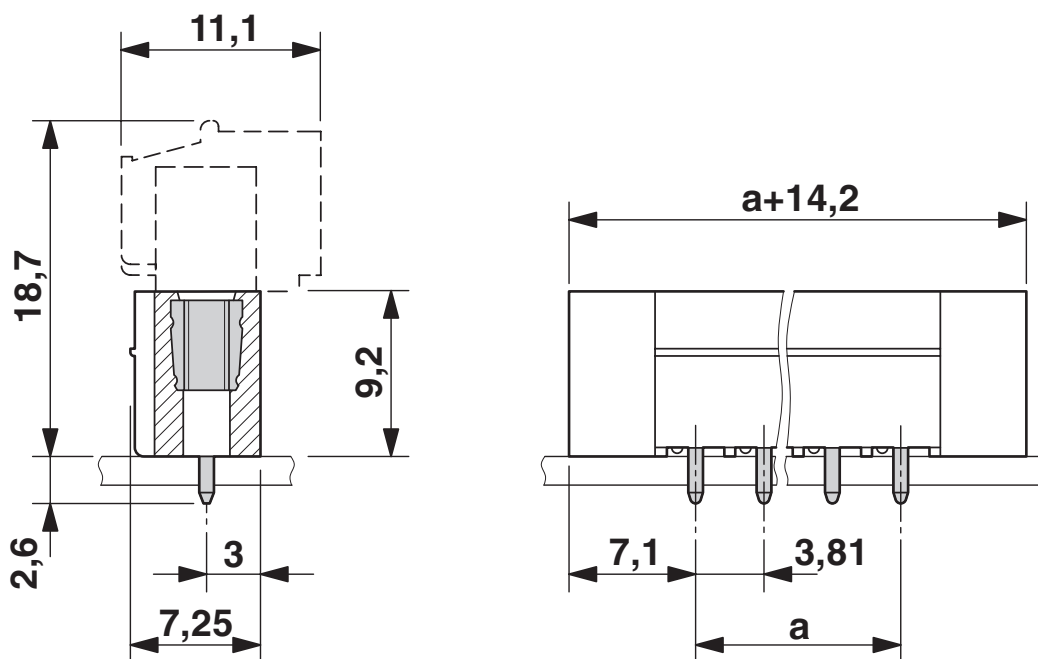
Rysunek wymiarowy
