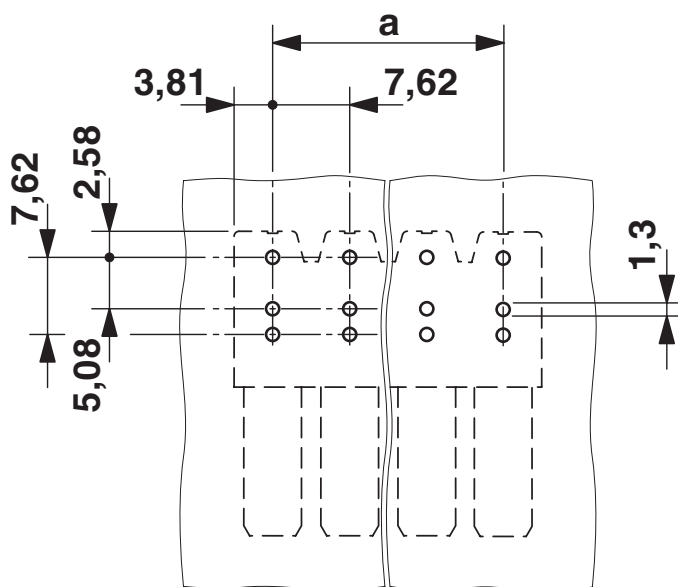
Otworowanie/geometria płytek lutowniczych
