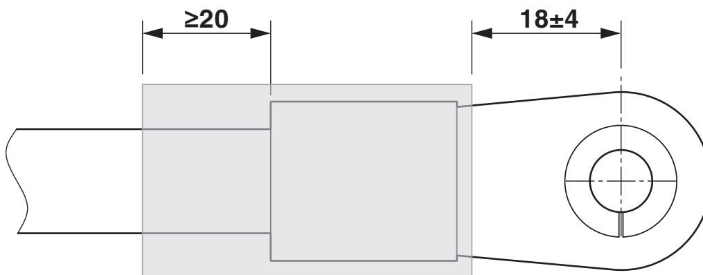
Rysunek wymiarowy
