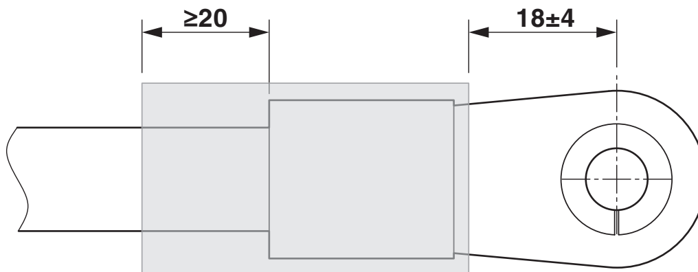
Rysunek wymiarowy
