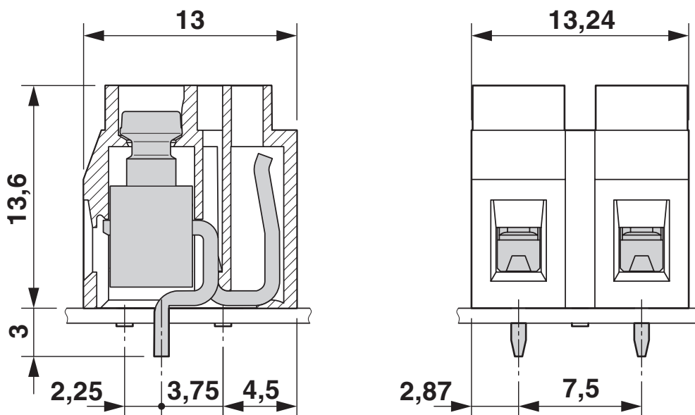
Rysunek wymiarowy
