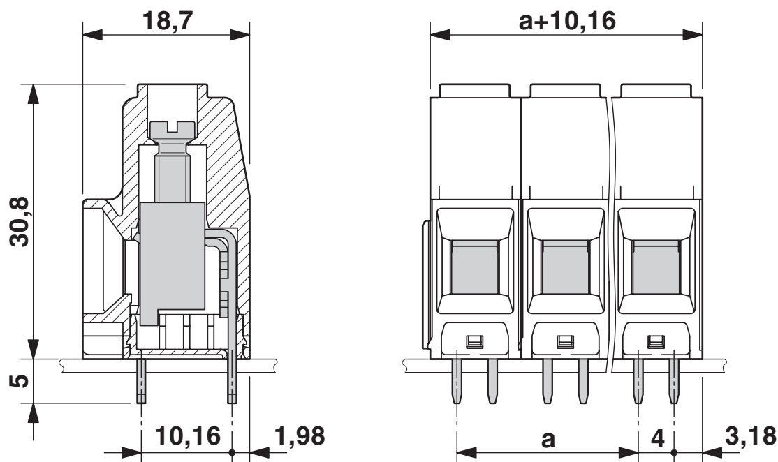
Rysunek wymiarowy
