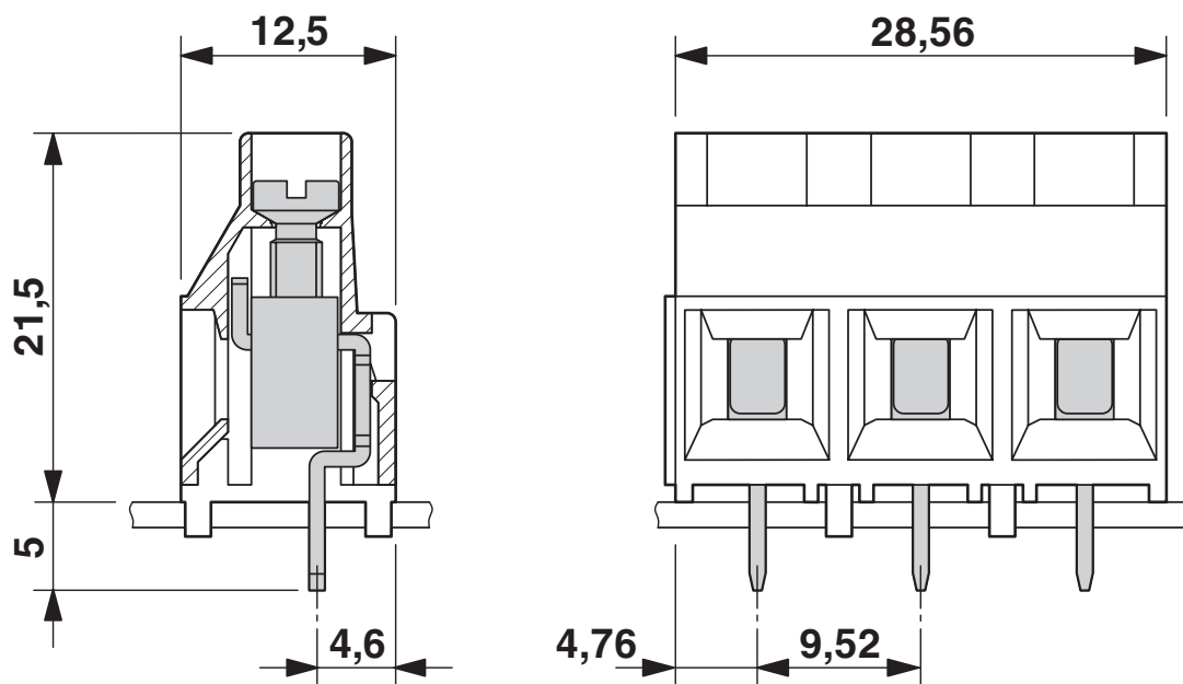
Rysunek wymiarowy
