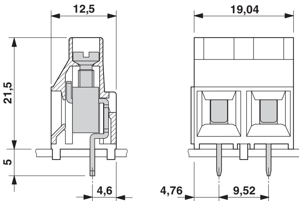
Rysunek wymiarowy
