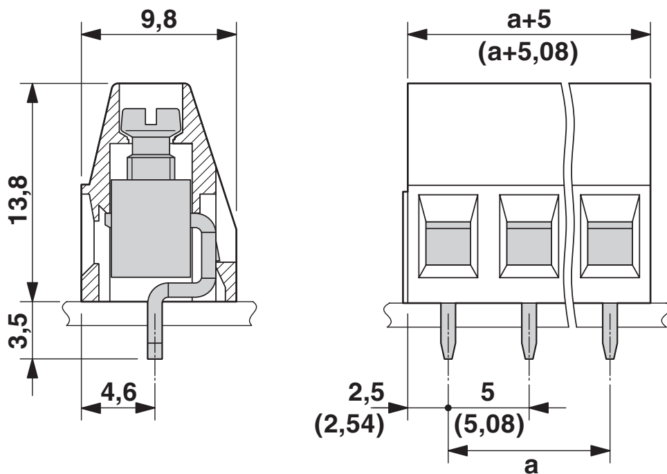
Rysunek wymiarowy
