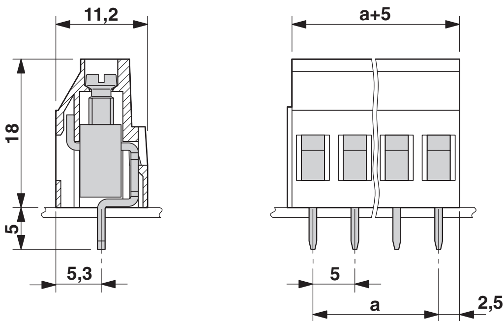
Rysunek wymiarowy
