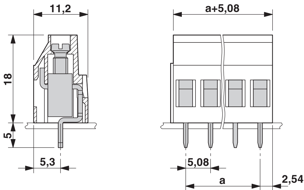
Rysunek wymiarowy
