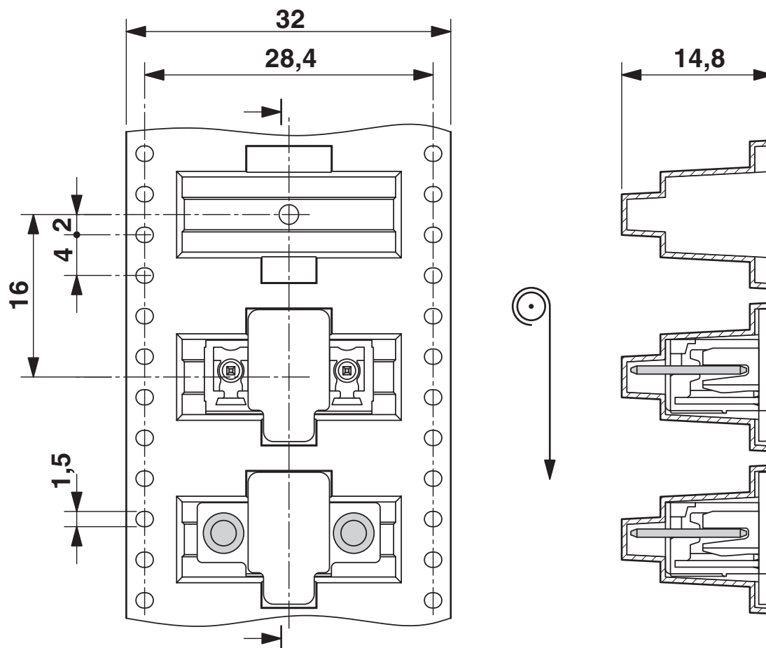
Rysunek wymiarowy
