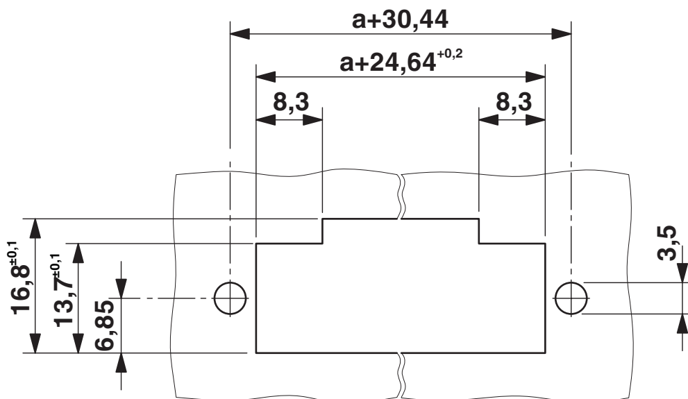
Rysunek wymiarowy
