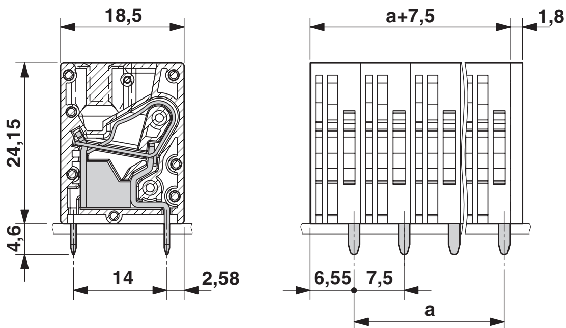
Rysunek wymiarowy
