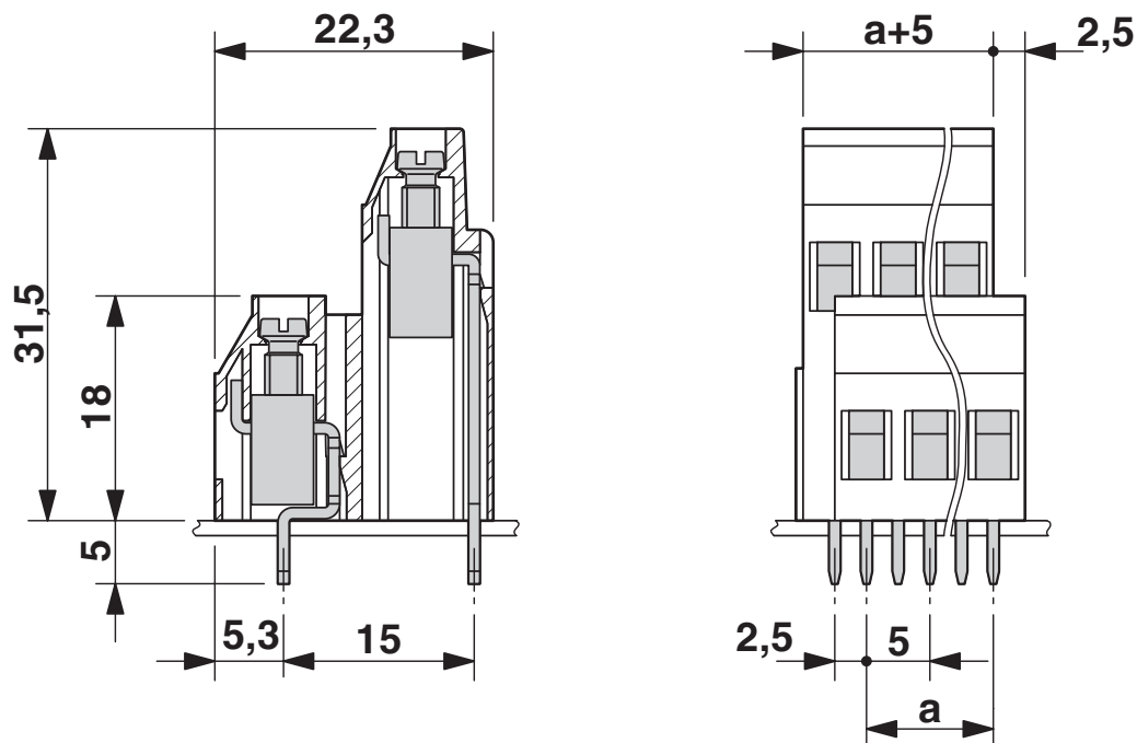
Rysunek wymiarowy
