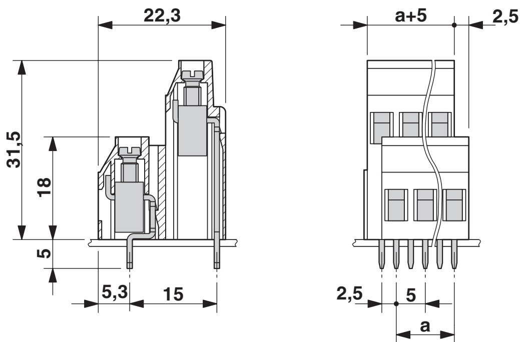
Rysunek wymiarowy
