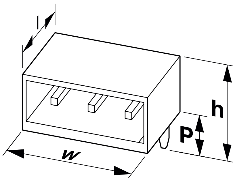
Rysunek wymiarowy
