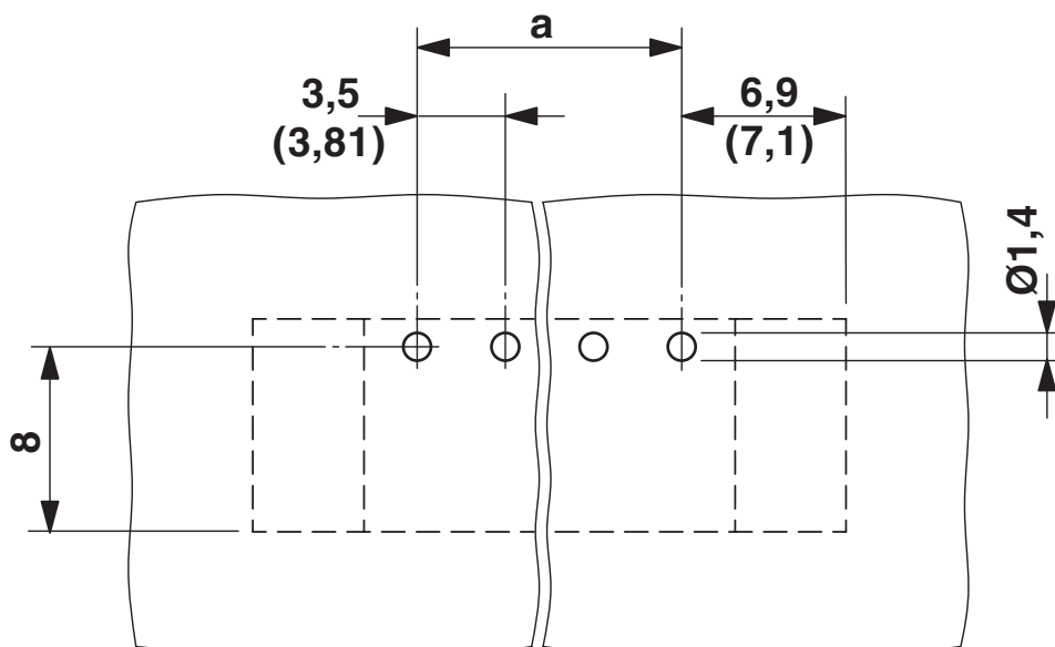
Otworowanie/geometria płytek lutowicznych
