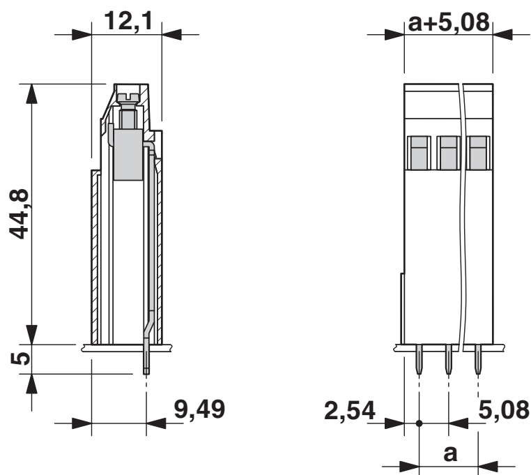
Rysunek wymiarowy wersji 3-biegunowej produktu
