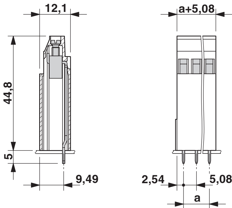
Rysunek wymiarowy
