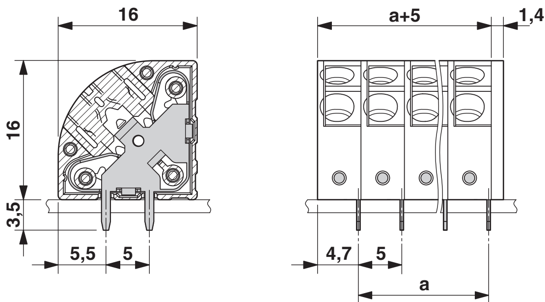
Rysunek wymiarowy
