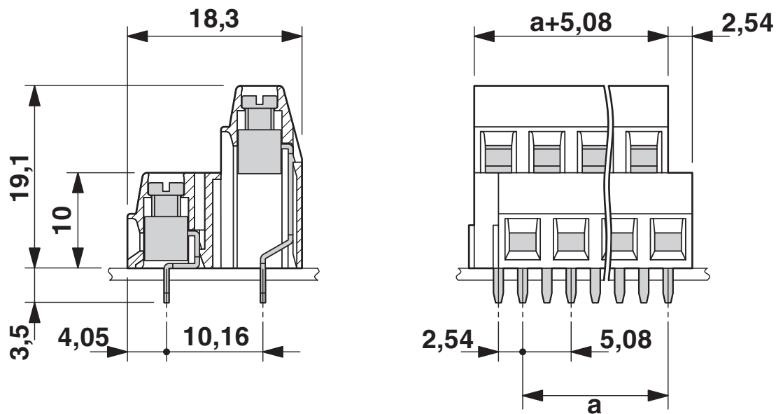
Rysunek wymiarowy
