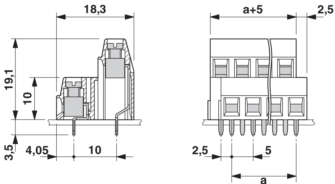
Rysunek wymiarowy
