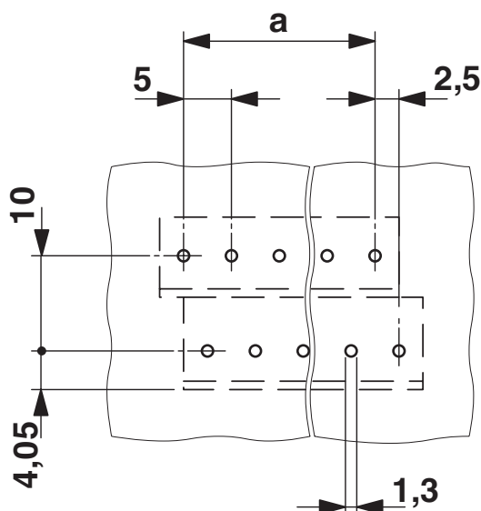
Otworowanie/geometria płytek lutowniczych
