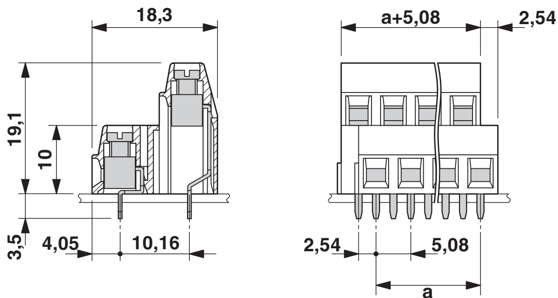
Rysunek wymiarowy
