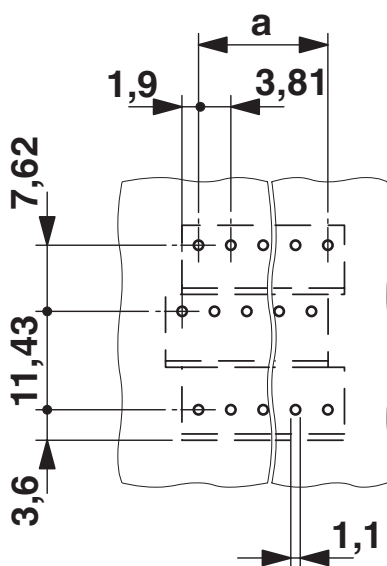
Otworowanie/geometria płytek lutowniczych
