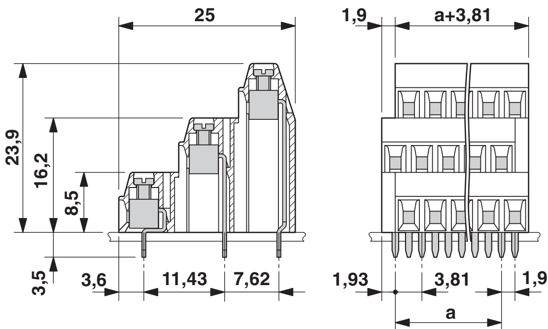
Rysunek wymiarowy
