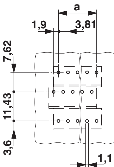
Rysunek wymiarowy
