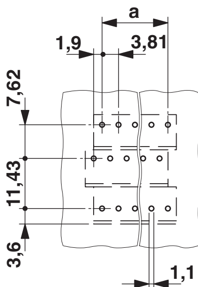
Otworowanie/geometria płytek lutowniczych
