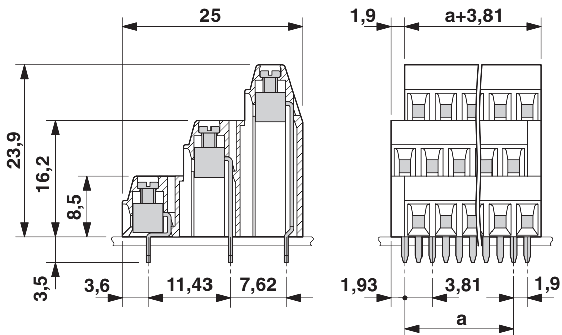
Rysunek wymiarowy
