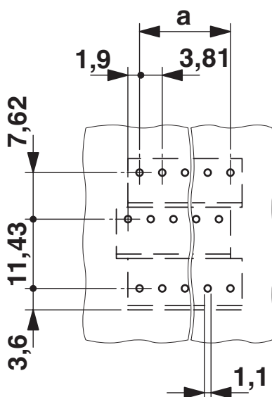
Otworowanie/geometria płytek lutowniczych
