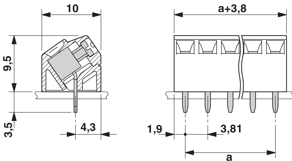
Rysunek wymiarowy
