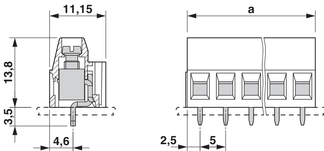
Rysunek wymiarowy
