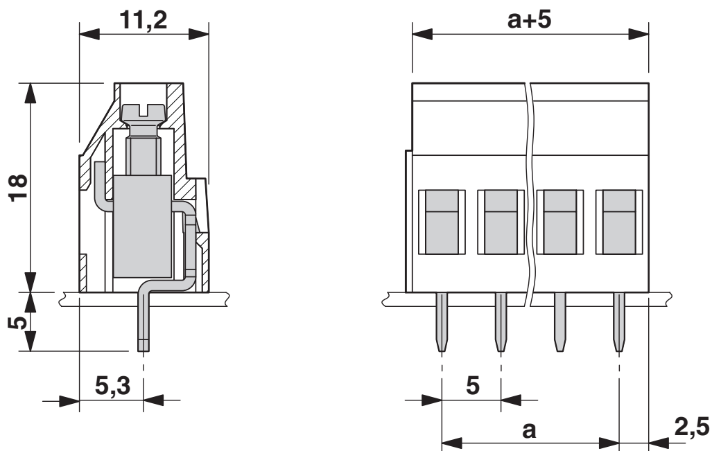
Rysunek wymiarowy
