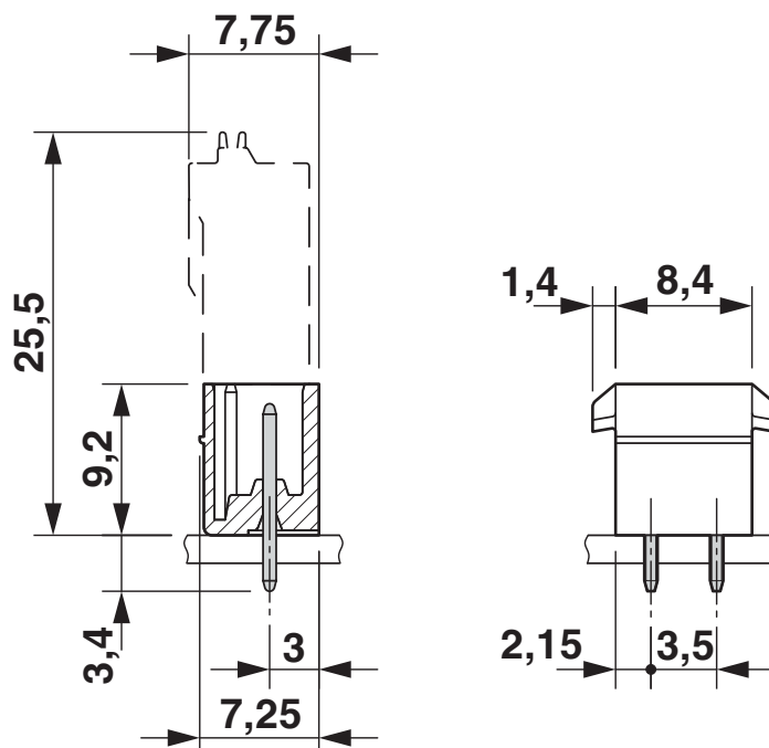
Rysunek wymiarowy
