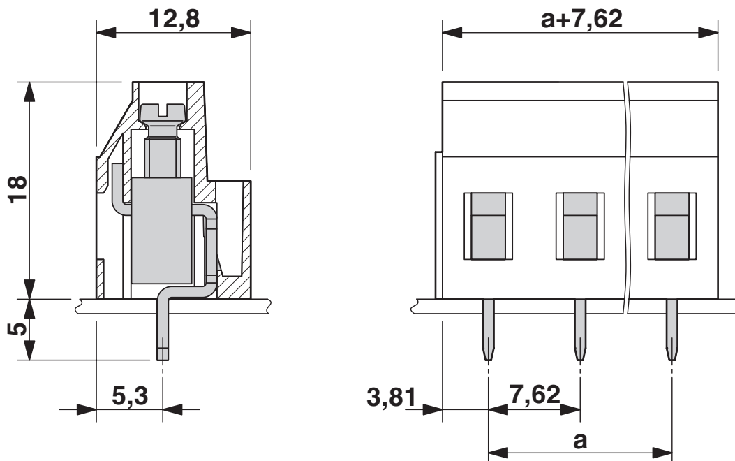
Rysunek wymiarowy
